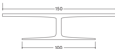
Telaio particolare: Telaio a T (vedi immagine)
